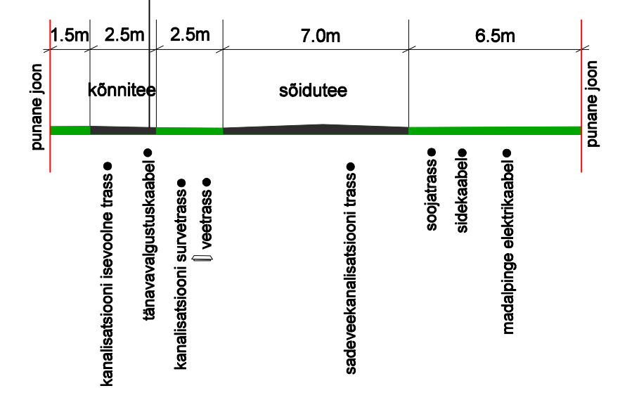
LÕIGE C-C'
