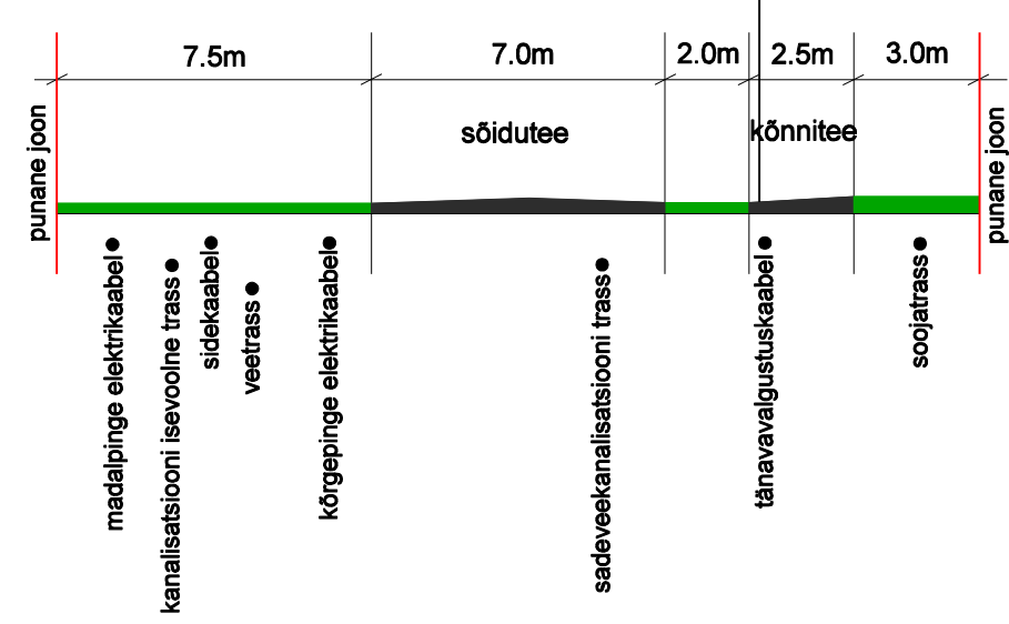
LÕIGE F-F'
