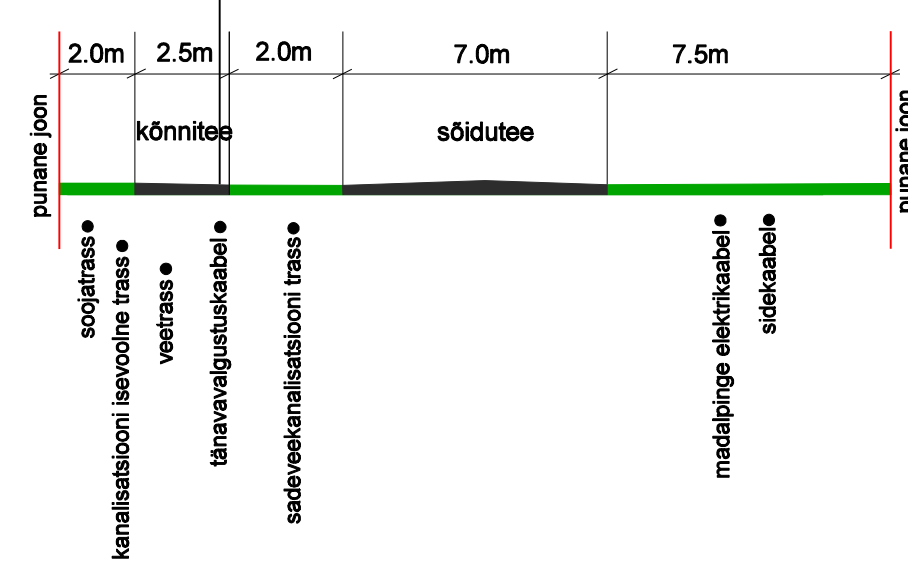
LÕIGE E-E'
