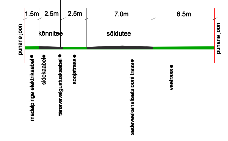
LÕIGE C-C'
