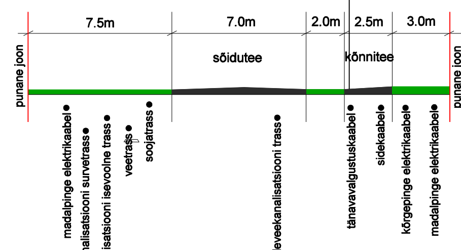
LÕIGE B-B'
