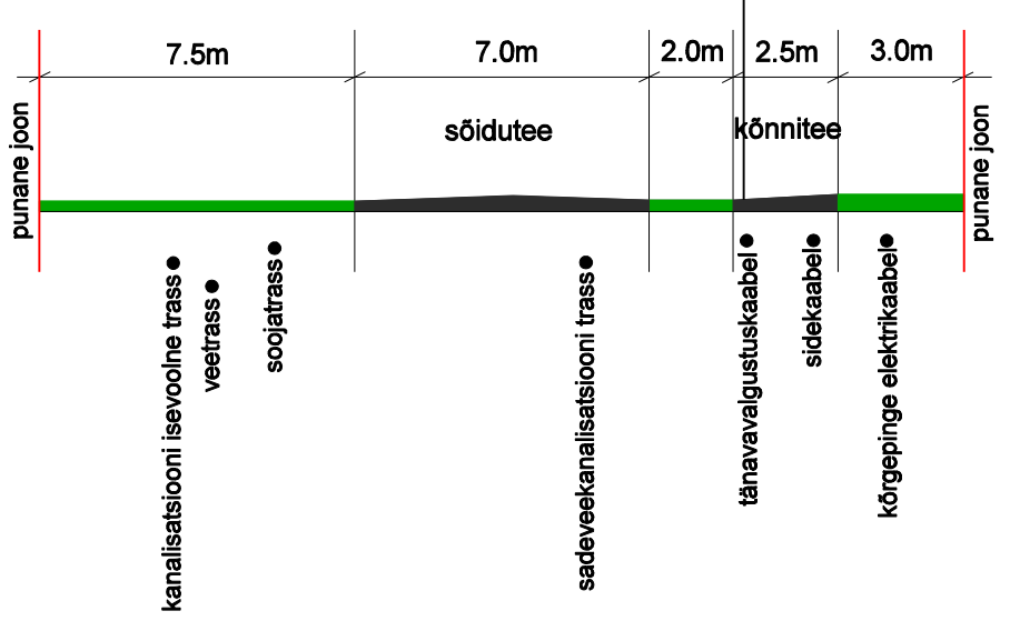
LÕIGE E-E'
